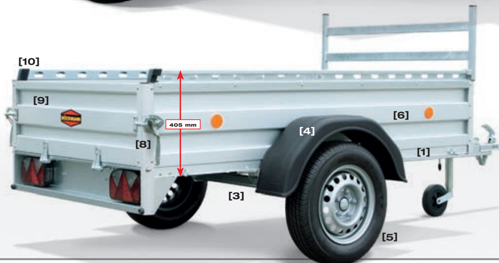
Abbildung: TL-AL 2111/10 Aluminium-Kastenanhänger, Einachser-Modell, ungebremselt, mit Stirn- und Seitenwandgalerie (Zubehör), Stützrad (Zubehör)
