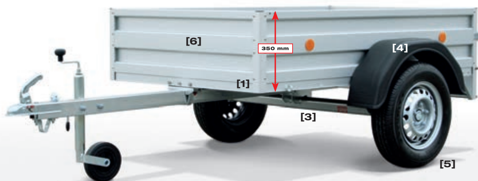
Abbildung: TL-AL 2111/75 Aluminium-Kastenanhänger, Einachser-Modell, ungebremst, Stützrad (Zubehör)
